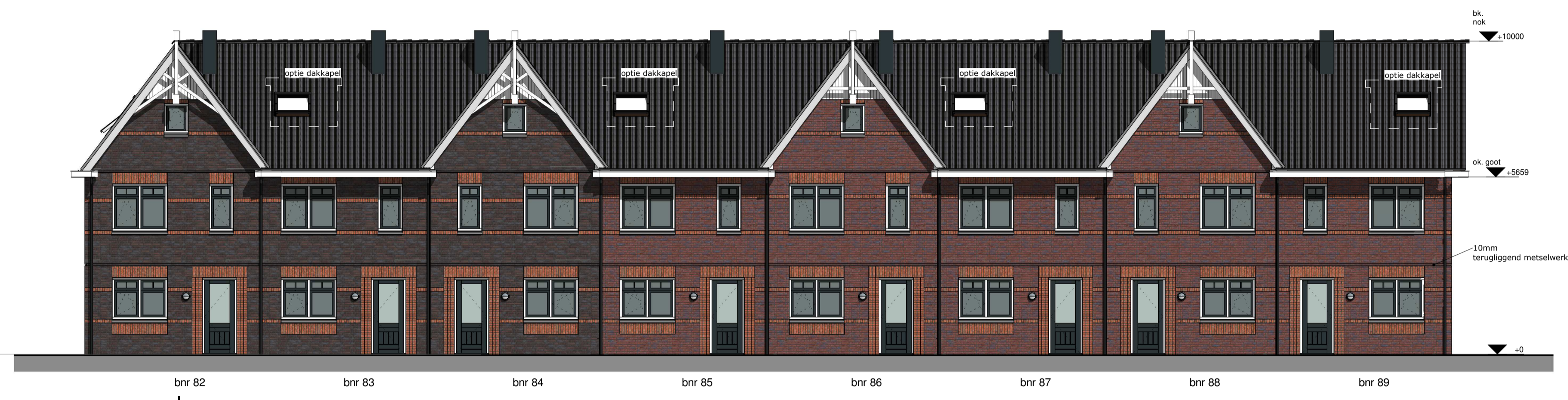
voorgevel
